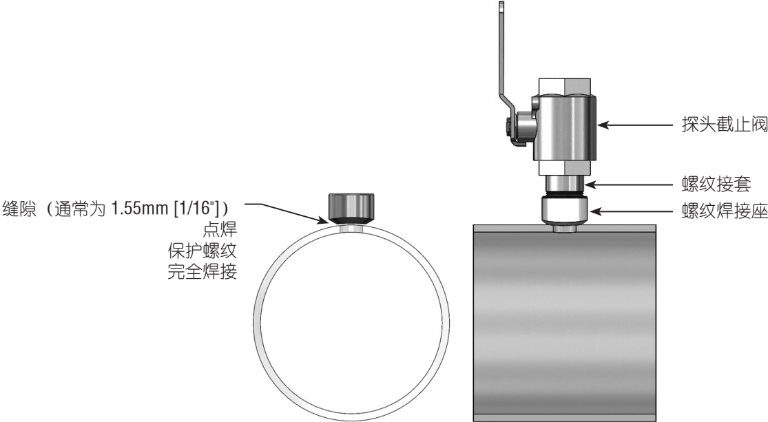
图 4.焊接缝隙
