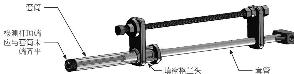
图 3. 套筒
